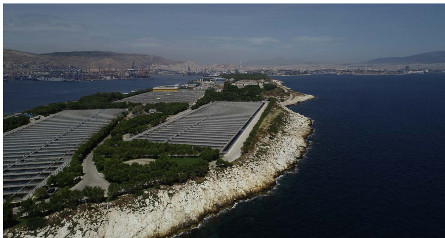
Κέντρο Επεξεργασίας Λυμάτων Ψυττάλειας (ΠΗΓΗ: ΕΥΔΑΠ)
